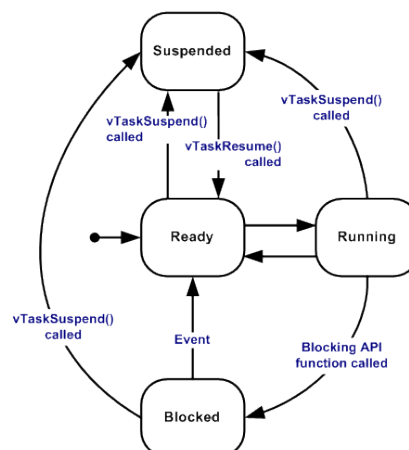
Abbildung 2: Die vier Task-Zustände im FreeRTOS-Scheduler.
