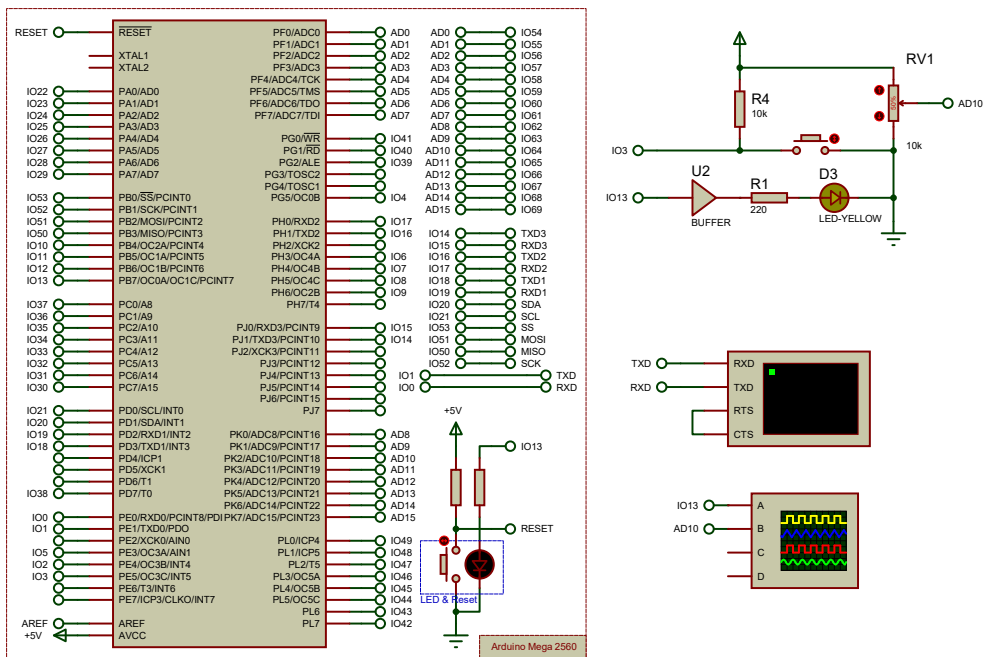
Abbildung 6: Schematic des Proteus Template Projektes (ue2-template2.pdsprj)
