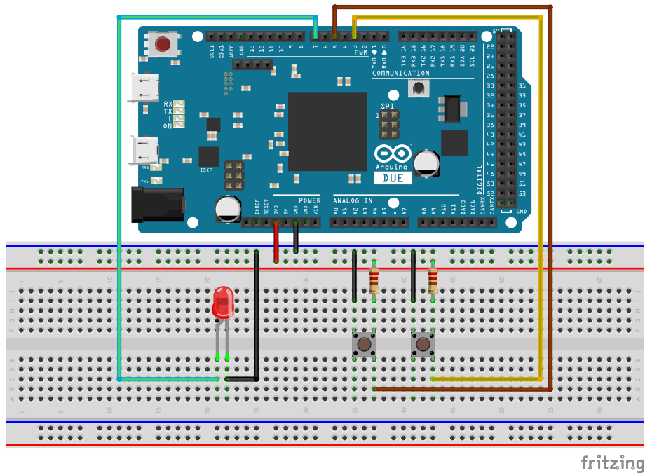
Abbildung 1: Vorschlag für die Verdrahtung des Versuchsaufbaus.
