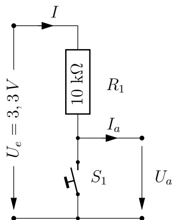
Abbildung 2: Taster mit Pullup-Widerstand
