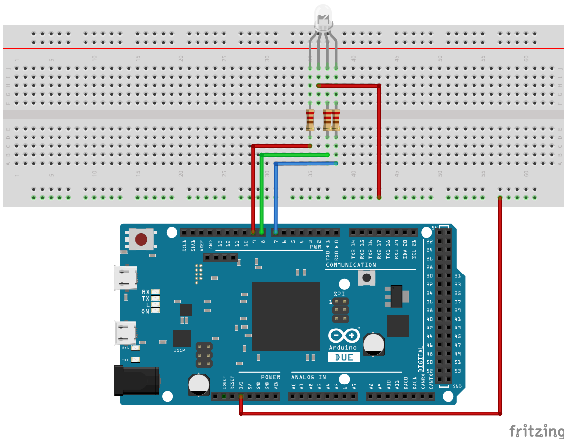
Abbildung 1: Vorschlag für die Verdrahtung des Versuchsaufbaus.
